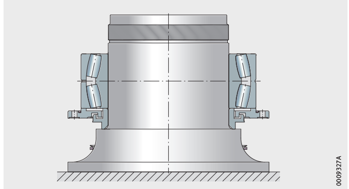
图 11 轴承的安装
