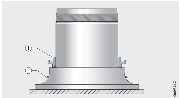
图 9 安装叶轮侧迷宫密封圈
