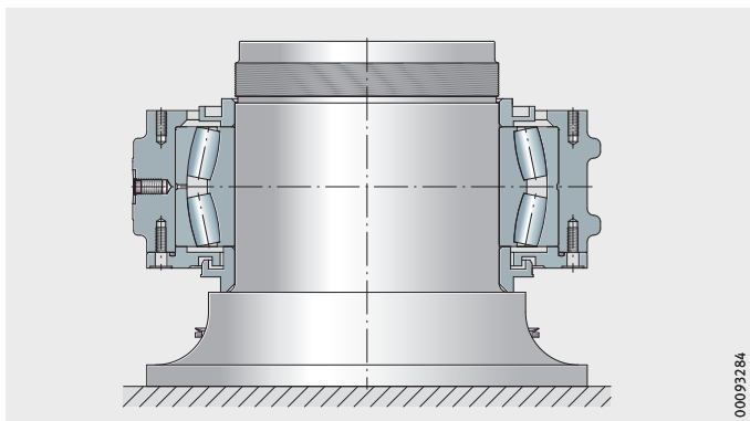
图 13 齿轮箱侧迷宫式密封环的安装
